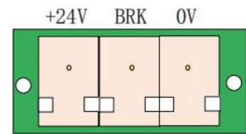
图2.3 欧规端子插座
