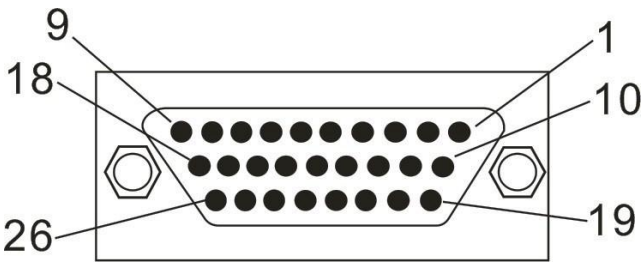
图 2.5 三排DB26母座
