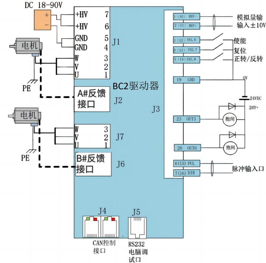
BC2系列系统接线图
